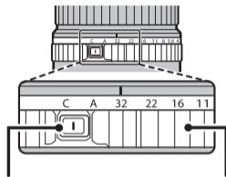
Przycisk zwolnienia blokady pierścienia przysłony Pierścień przysłony
