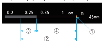
Отображение фокусного расстояния (изображение) телеобъектива
