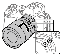
Позначки встановлення
